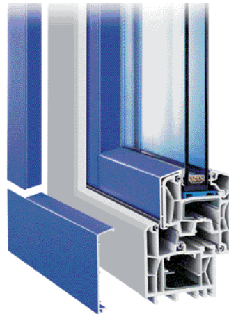
Modell hilzinger Innotherm-Alucolor, System Mitteldichtung, 70mm Bautiefe, flächenversetzt mit lichtgrauen Dichtungen und äußerer Aluminiumschale.
