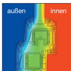
Die Wärmebildaufnahme zeigt den optimierten Wärmeverlauf des Fenstermodells hilzinger Prestige.
