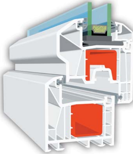
Modell hilzinger Prestige, System Anschlagdichtung, halbflächenversetzt mit Stillflügel im äußeren Bereich des Fensterflügels.
