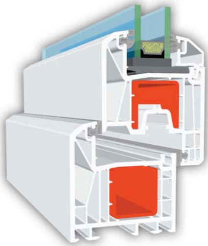
Modell hilzinger Prestige, System Anschlagdichtung, flächenversetzt mit harmonisch abgerundeten Konturen und lichtgrauen Dichtungen.
