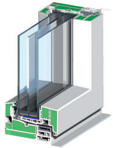
VADB-plus Passivhausfenster
