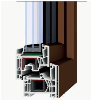
hilzinger Zenit 76 AluClip in der schlanken Standardausführung 3) mit 74 mm Rahmenansicht.
