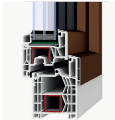
Ausführung mit breitem Rahmen in der Ansichtsbreite 104 mm und AluClip Kurzschale, z.B. geeignet in Verbindung mit dem Einsatz eines Wärmedämmverbundsystems. Optional auch in der Rahmenansichtsbreite 92 mm erhältlich.
