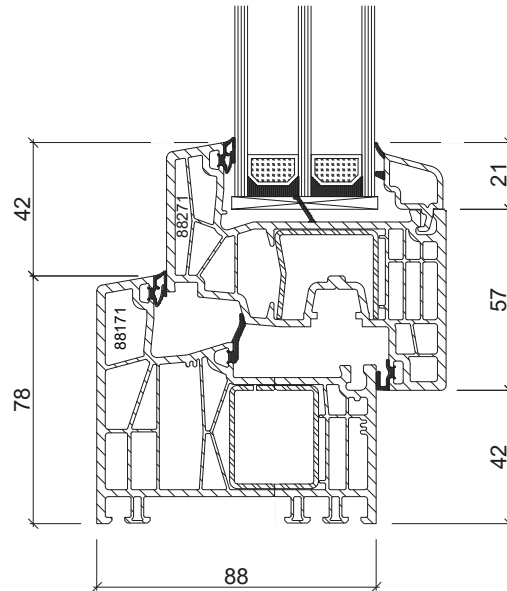
Master 88 Standardrahmenansicht 78 mm weiß
